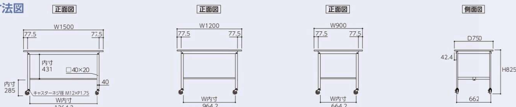
SLKC-1575TT-BKW 75φ自在ストッパー付ゴムキャスター 4個
