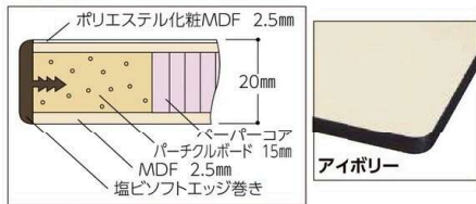
SWPW-2412-II使用例
