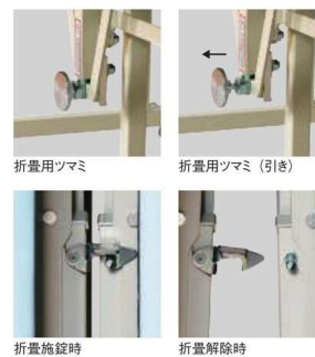
安全ロック
