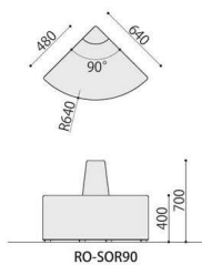
RO-SOR90
