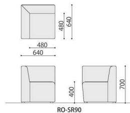
RO-SR90
