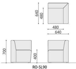
RO-SL90
