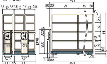
標準寸法
