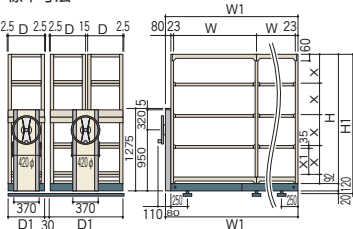
呼び寸法H2100×W1460×D300 天地6段
