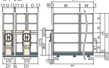
呼び寸法H2100×W1500×D300 天地6段
