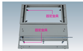
床固定金具 SFS-A P417
