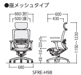
4軸シンクロロック機構 クラス最大の傾動範囲を実現したシンクロロック機構は、アルミ合金フレームにより背30°・座10°のダイナミックな動きを採用。ダイナミックな4軸メカとサスペンション・ファブリックが体を心地良くホールドします。また、ロックングストッパーによりベストポジションでの快適なパソコン作業をサポートします。
