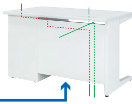
①アース付2口コンセント ②LANジャックホルダー
