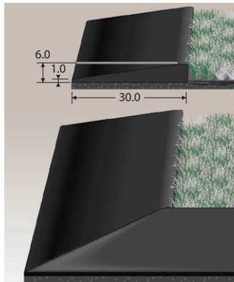
傾斜タイプ 断面イメージ図
