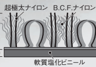
断面形状
