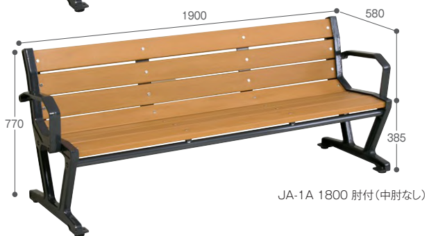
JA-1 1800 肘なし(中肘なし)
