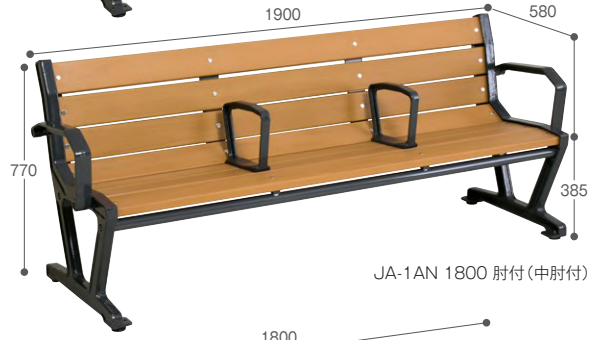
JA-1N 1800 肘なし(中肘付)
