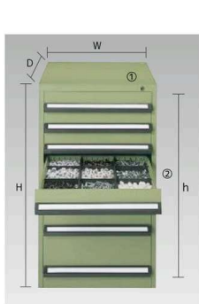
H800 外寸法/W580xD600xH800mm
